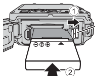
Защелка батареи
