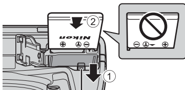
Защелка батареи
