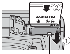
Akkusalpa
