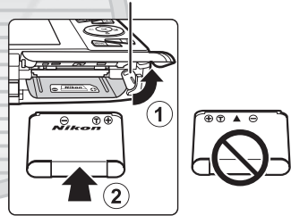
Pil mandalı
