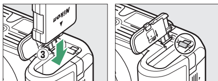
电池锁门
