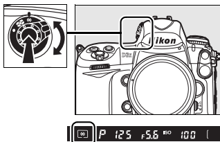
Selector de la medición
