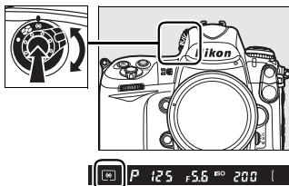
Botón de bloqueo del selector de la medición
