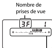
Nombre de prises de vue Écran de contrôle Indicateur de bracketing de la balance des blancs
