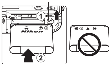
Blocco batteria
