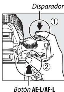
Botón AE-L/AF-L
