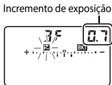
Incremento de exposição Panel de controlo secundário
