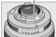
CPU 镜头
